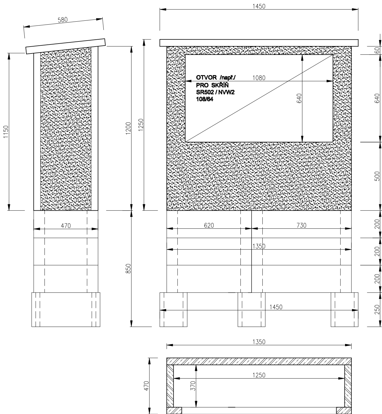
SKŘÍŇ ELEKTRO SR135
