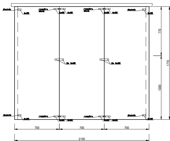
Montážní pohled na zadní díly
