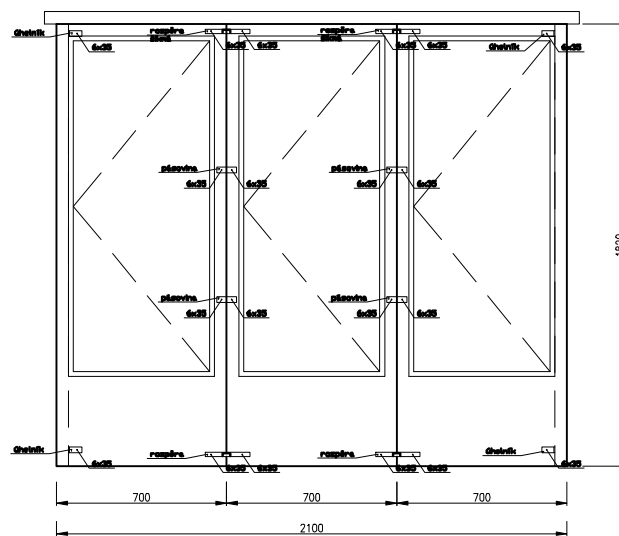
Montážní pohled na přední díly
