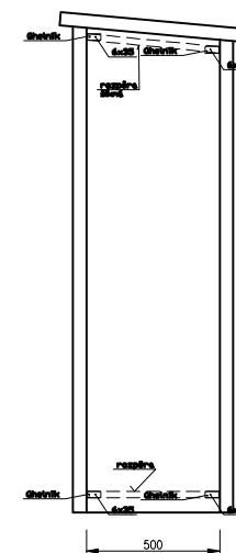
Montážní pohled na boční díl
