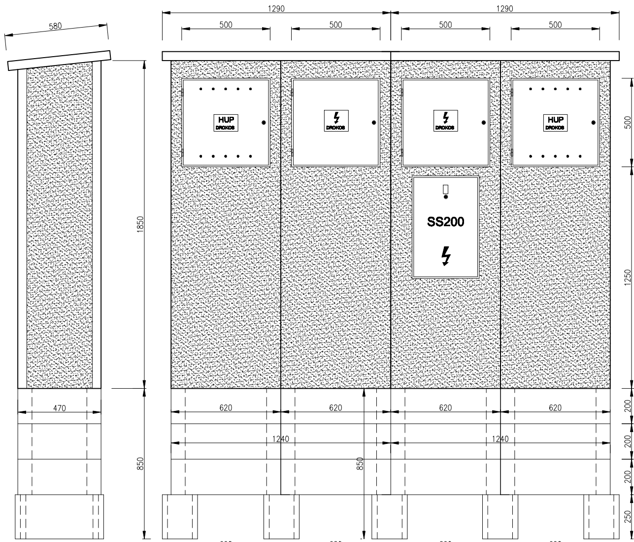
SESTAVA SKŘÍNÍ PLYN ELEKTRO PEV PRO DVA DOMY
